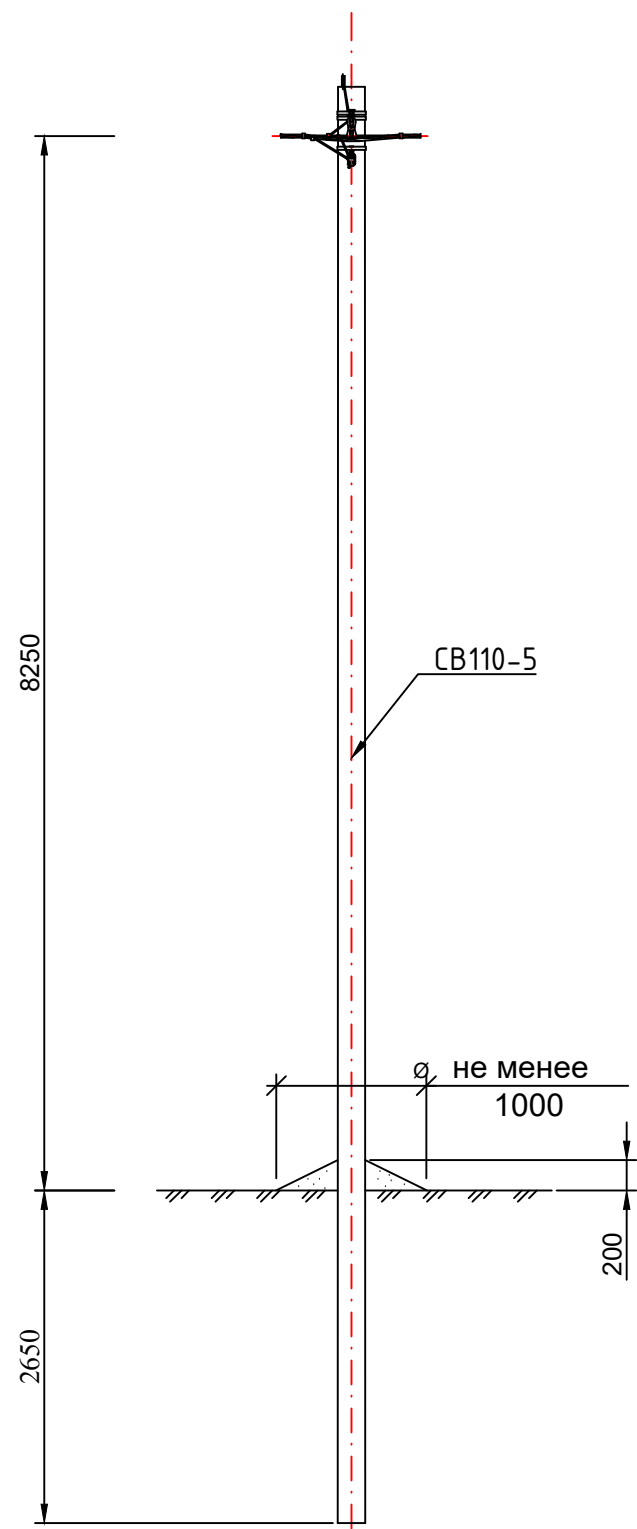
Схема установки стойки CB110-5 (промежуточная опора)
