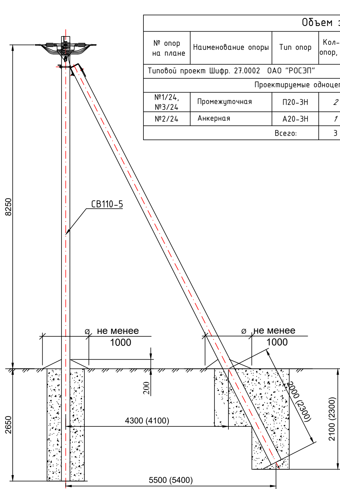
Схема установки стойки CB110-5 (анкерная опора)
